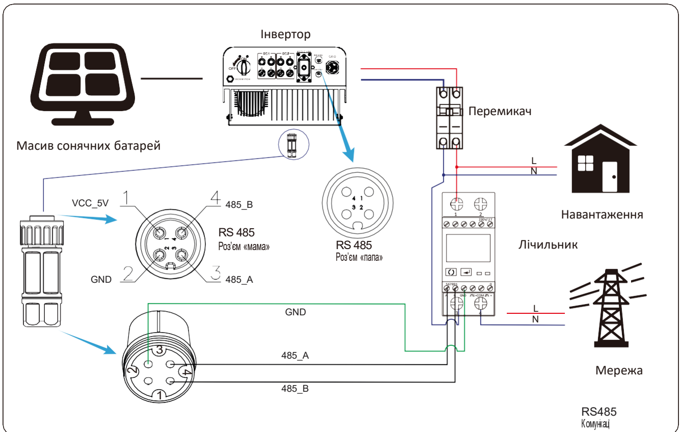
Мал.7.2. Схема підключення лічильника Eastron
