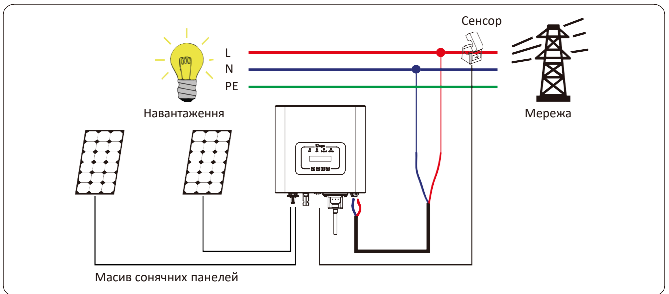
Мал.7.11. Схема підключення затискача датчика
