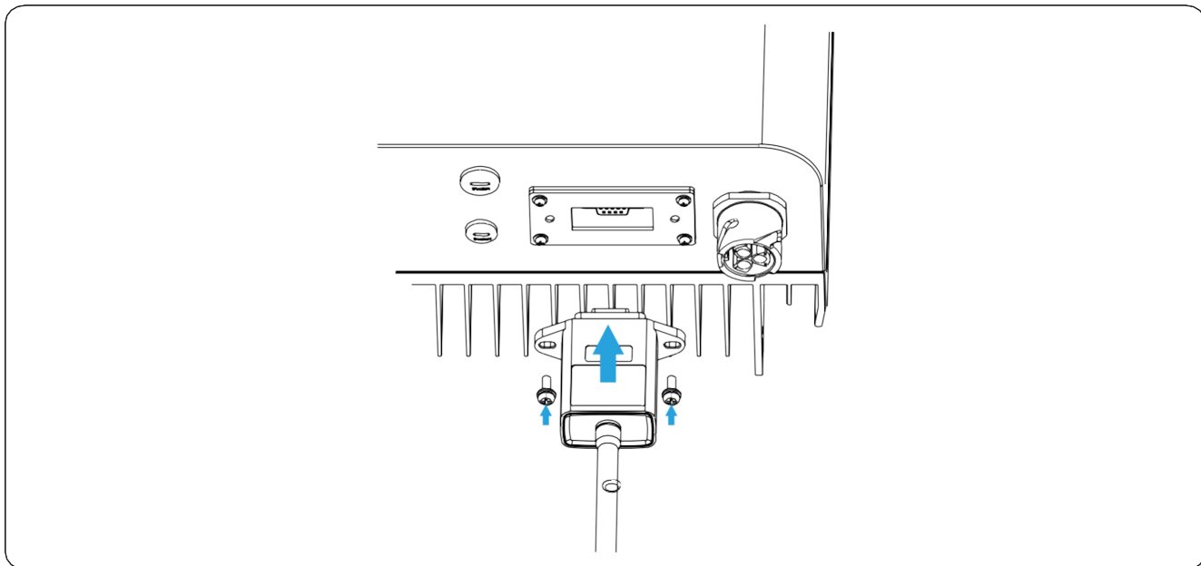
Мал.5.13. Підключення реєстратора даних
