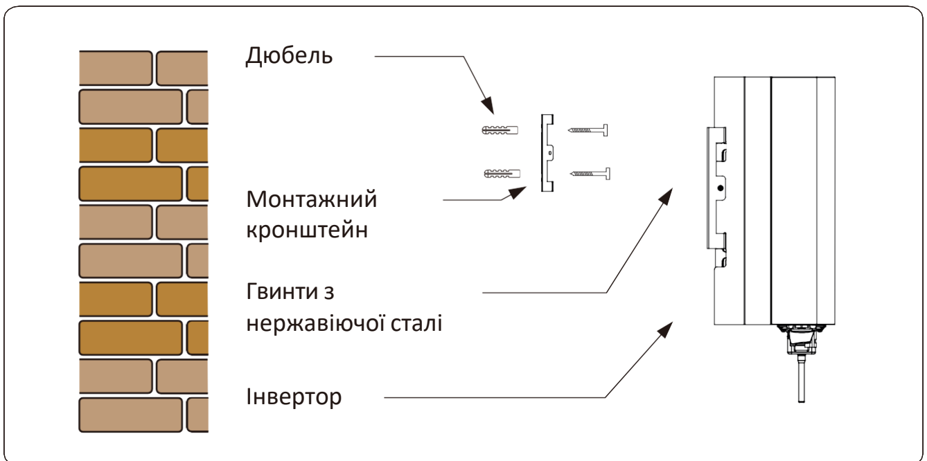
Мал.4.4. Установка інвертора
