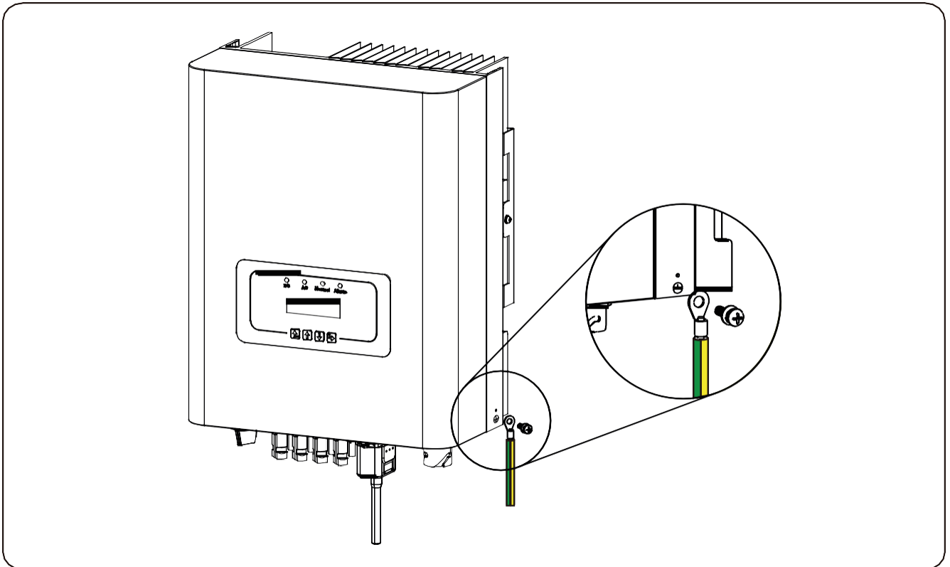
Мал.5.11. Монтаж заземлюючого проводу до корпусу
