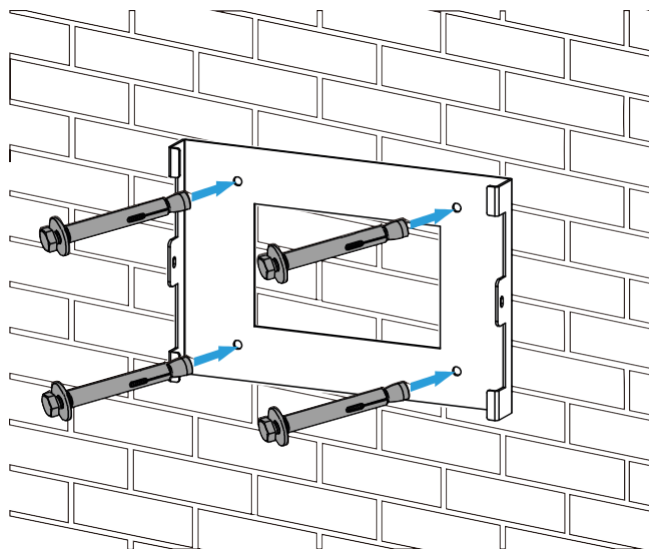
Мал.4.5. Монтаж кронштейна
