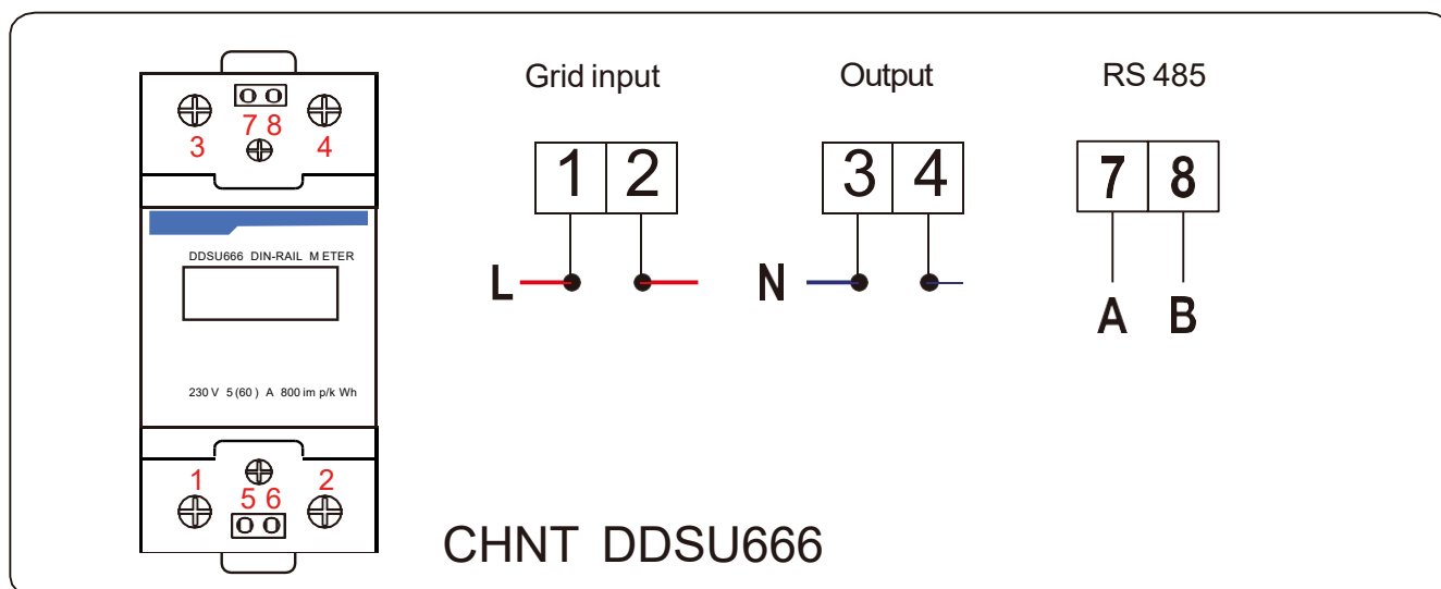
Мал.7.4. Лічильник CHNT
