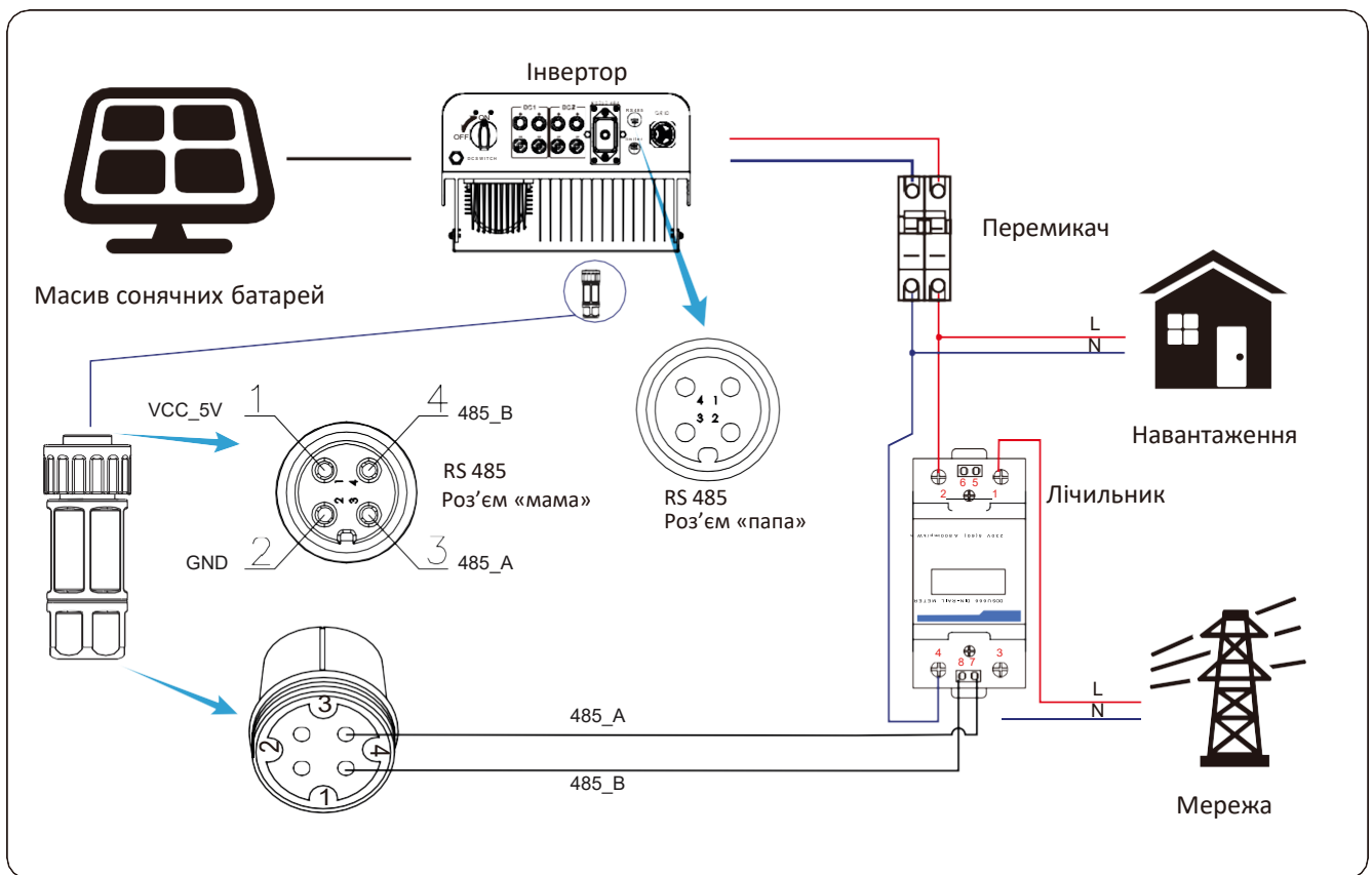
Мал.7.5. Схема підключення лічильника CHNT
