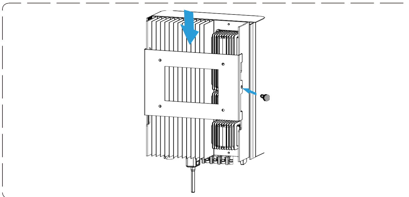
Мал.4.6. Установка інвертора
