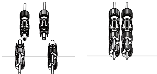
Мал. 3.6 Підключення входу постійного струму
