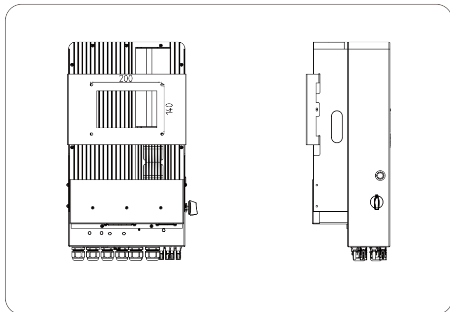
Розміри інвертора
