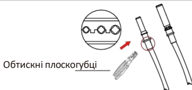
Мал. 3.4 Обтисніть контактний штифт до дроту
